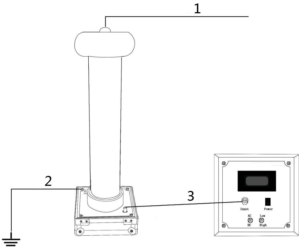
图 4 接线图
