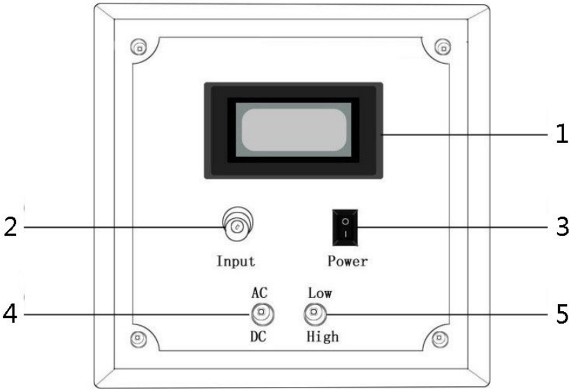
图 3 低压显示表
