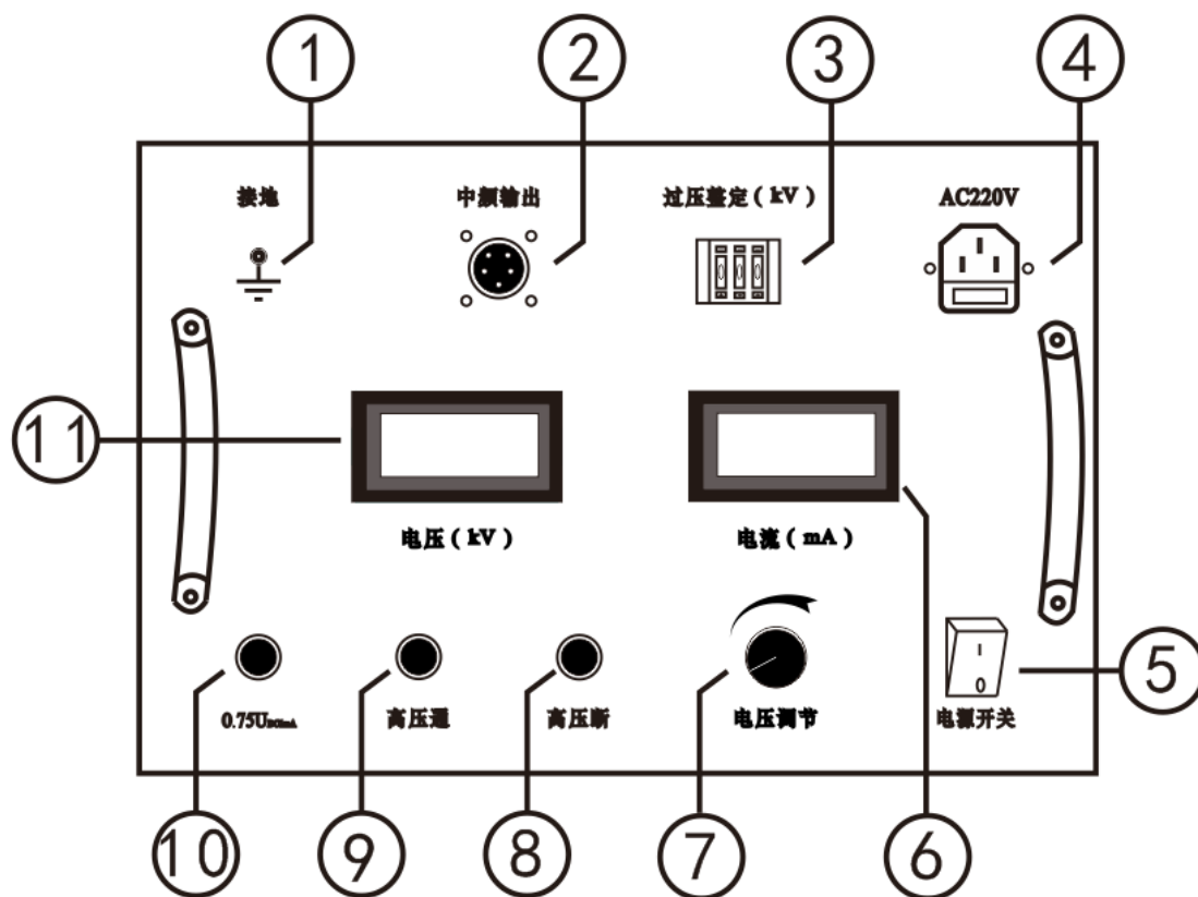
图 2 面板布局图
