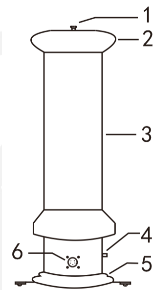
图 3 倍压筒示意图
